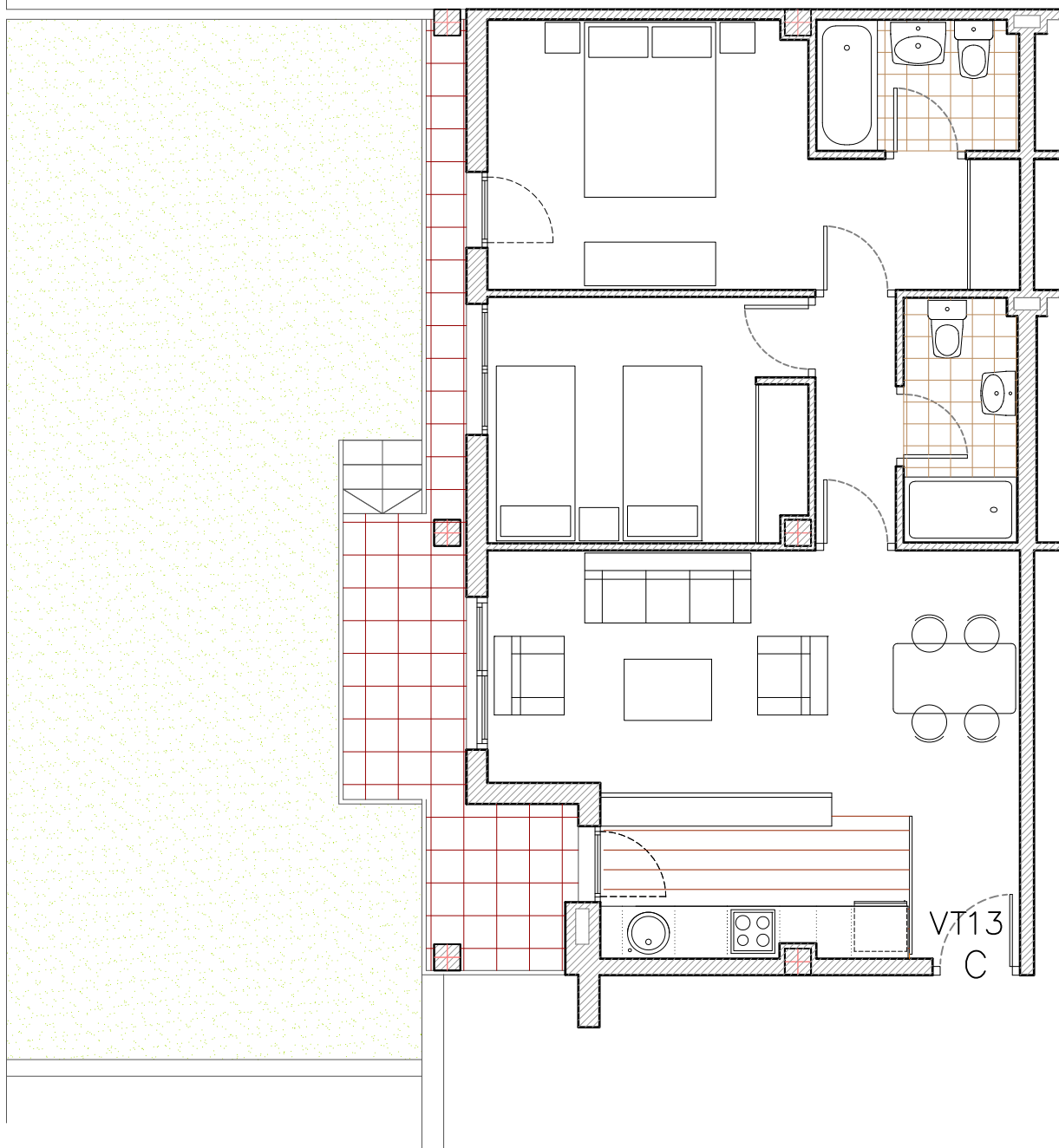
PLANTA BAJA
