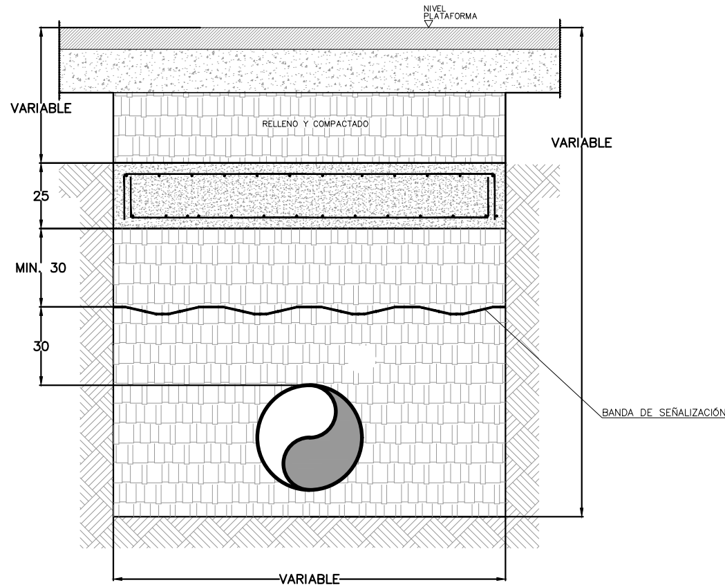
DETALLE TIPO SECCIÓN TRANSVERSAL
